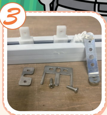
3 將軌道五金全部拆卸
